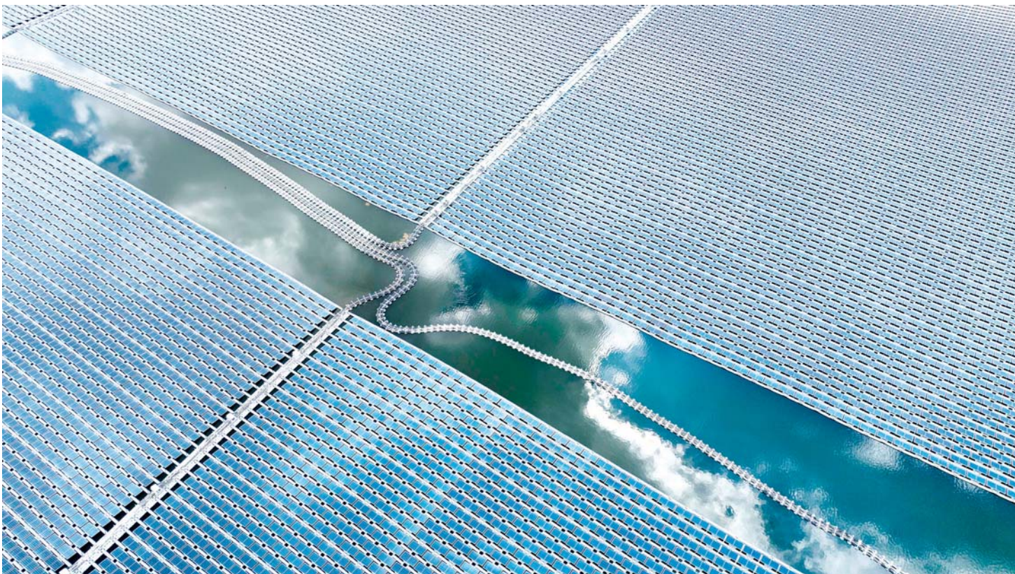
这是8月20日拍摄的位于宁夏灵武市马家滩镇的国家能源集团宁夏电力公司宁东电厂漂浮分布式光伏发电项目（无人机照片）。宁夏灵武市靠近沙漠、紧邻黄河，地处国家能源“金三角”核心区域，光源充裕，风能资源丰富。近年来，灵武市加快通过“光伏+”发电、风光互补发电、老旧风电场“以大代小”更新改造、分布式光伏规模化应用四种模式发展绿色能源产业，走上了绿色能源发展之路。截至2024年7月，灵武市新能源项目并网容量约394万千瓦。
